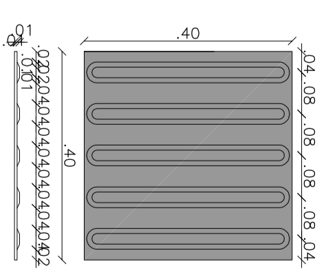
3 DETALHE PISO TÁTIL DIRECIONAL ESC.: 1:10
