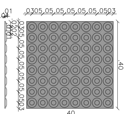
2 DETALHE PISO TÁTIL DE ALERTA ESC.: 1:10
